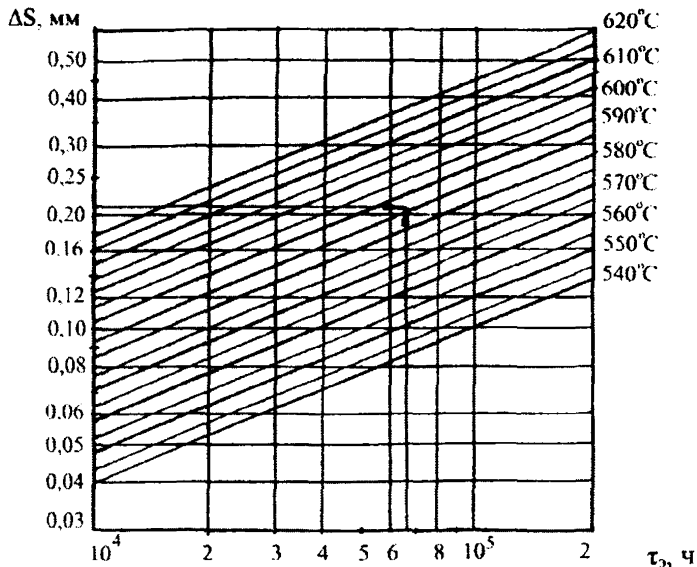
Рисунок 8.3. - График для определения эквивалентной температуры эксплуатации металла труб из стали 12X1МФ по глубине коррозии
